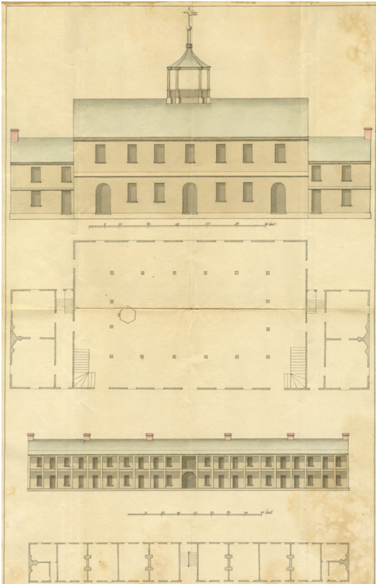
Projekt zabudowań szpitala w West Point, wyk. Tadeusz Kościuszko, 1779–1782, Alexander McDougall papers, The New York Historical Society
